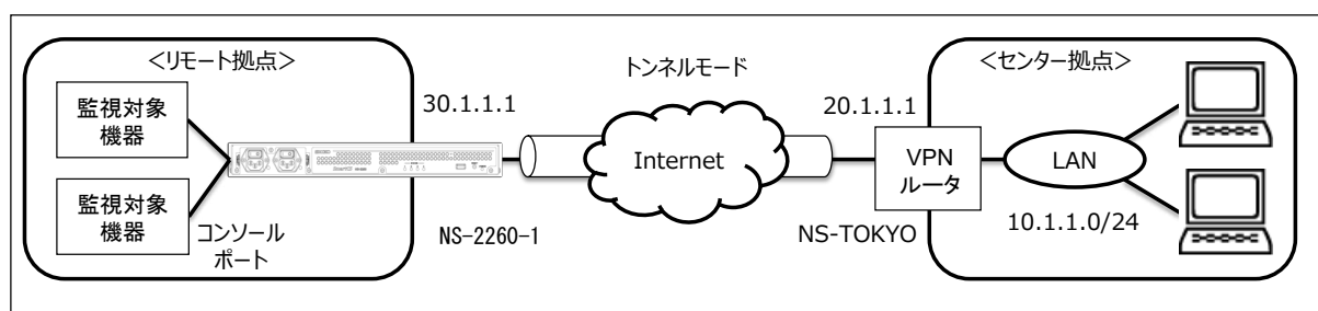
図 4-21 IPsec による VPN 構成
