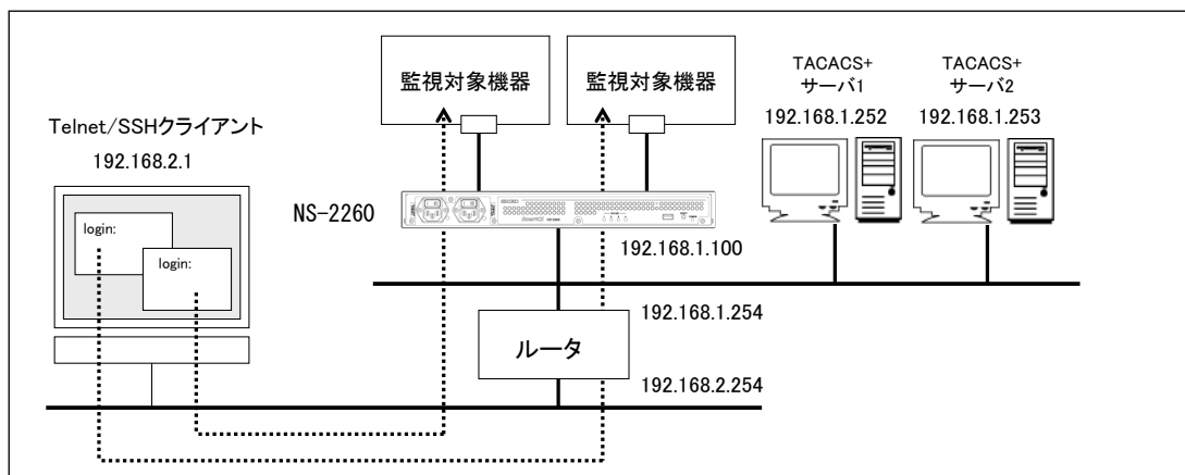
図 4-17 TACACS+機能 (基本構成)
