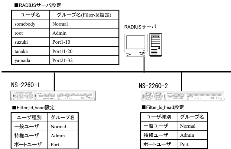
図 2-15 ユーザーグループの識別とシリアルポートのアクセス制限 (filter_id_head)
