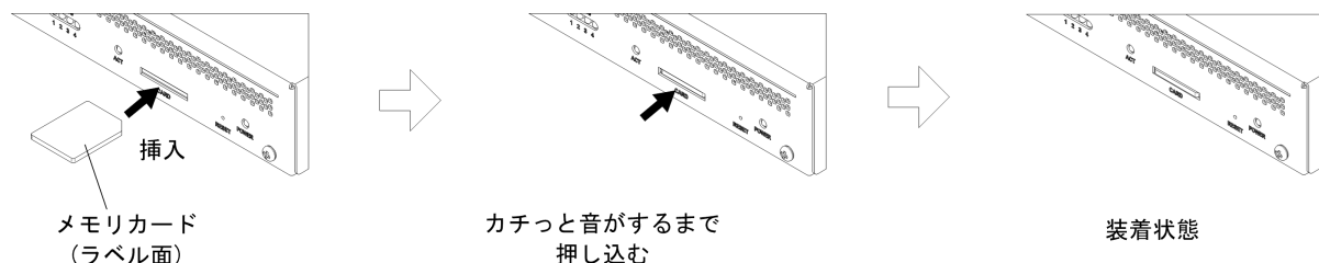
図 3-1 メモリーカードの挿入 (SmartCS)
