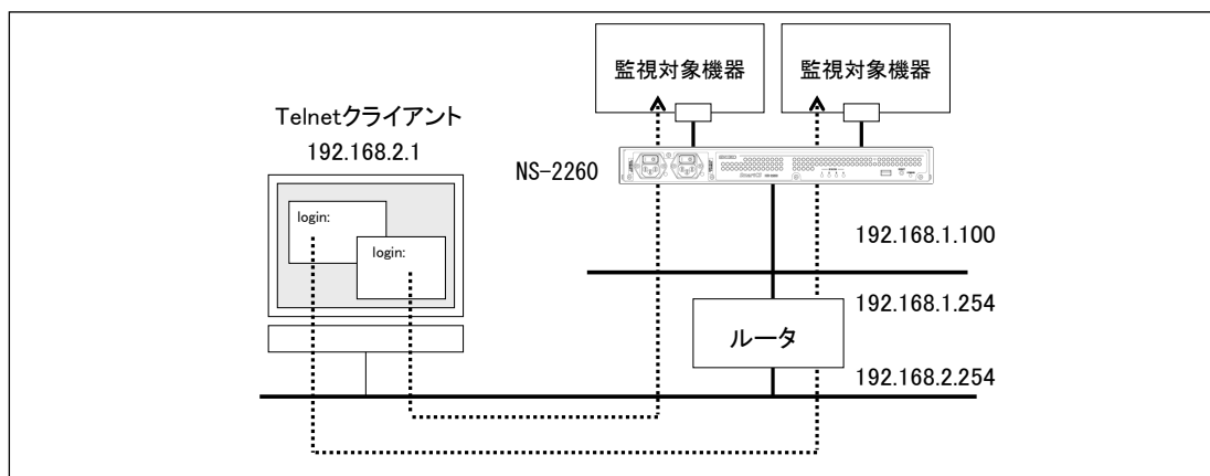
図 4-9 ポートログ保存機能の停止とポートサーバーメニューの表示の抑止
