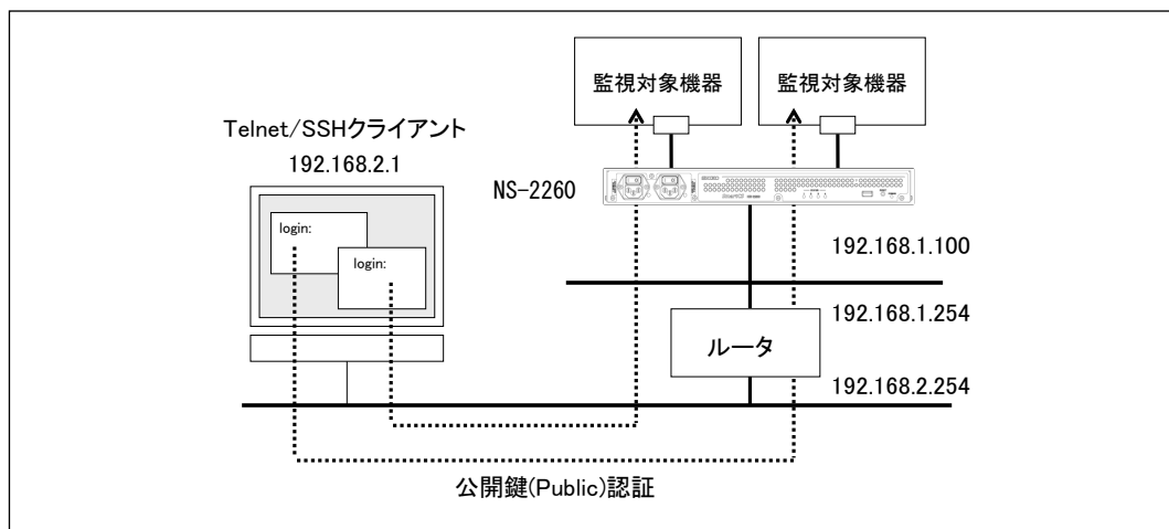
図 4-12 SSH 公開鍵 (Public) 認証
