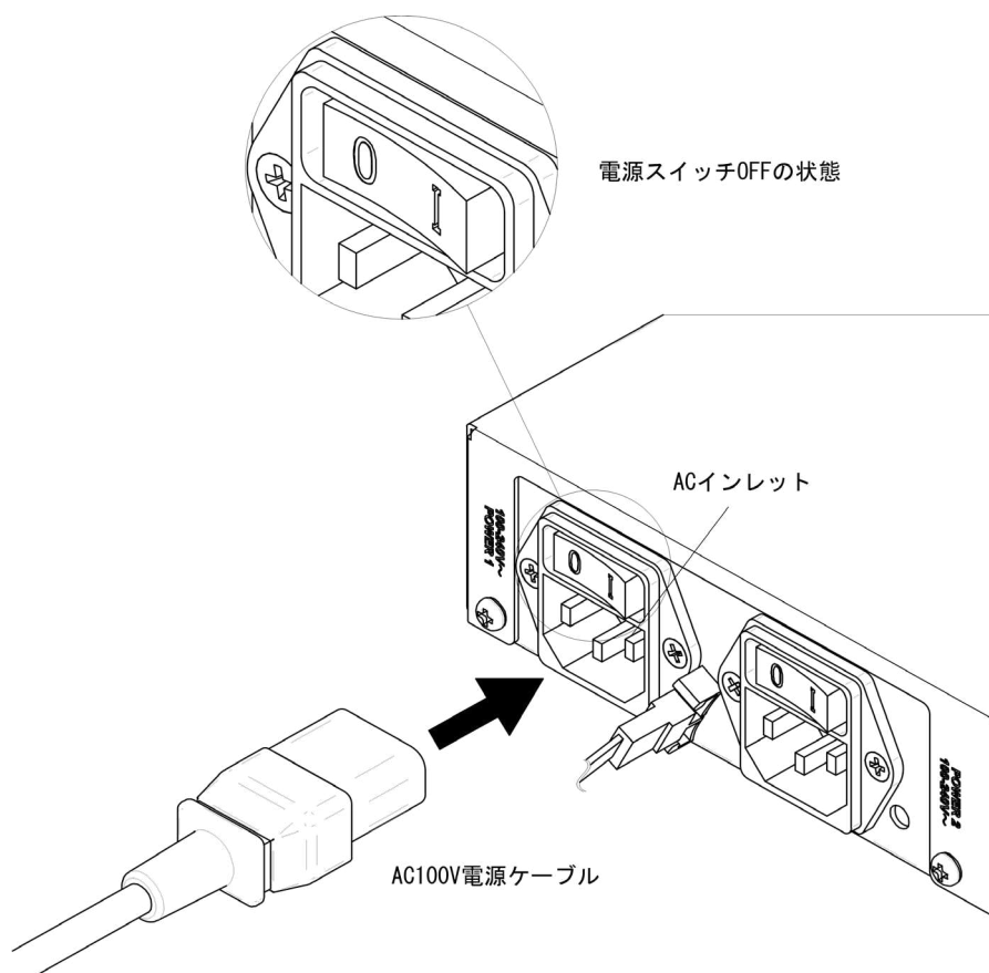
図 3-5 本装置の電源 ON
