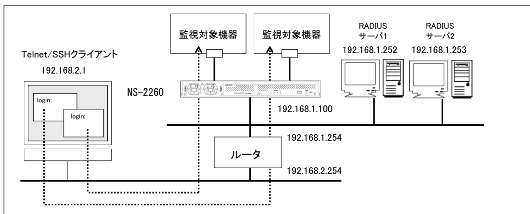
図 4-15 RADIUS 認証機能/RADIUS アカウント機能 (filter_id_head)
