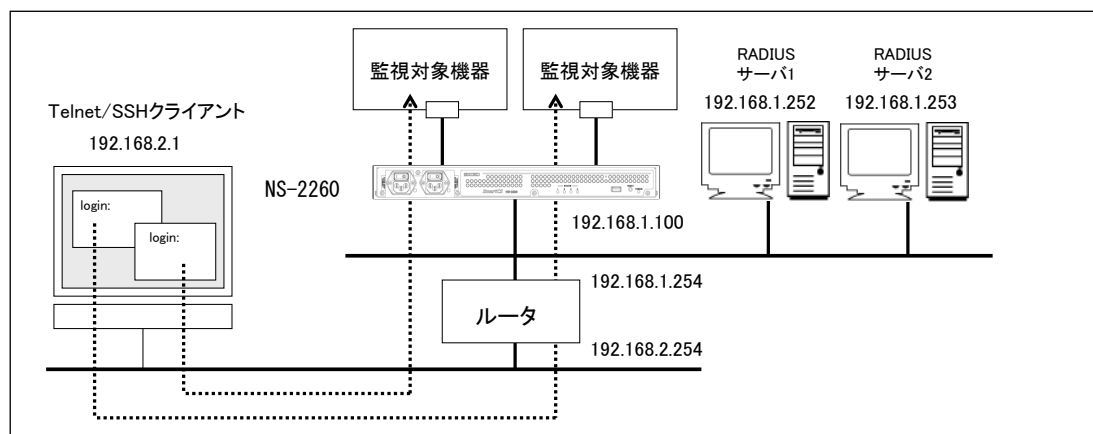
図 4-16 RADIUS 認証機能/RADIUS アカウント機能 (アクセスグループピンング)
