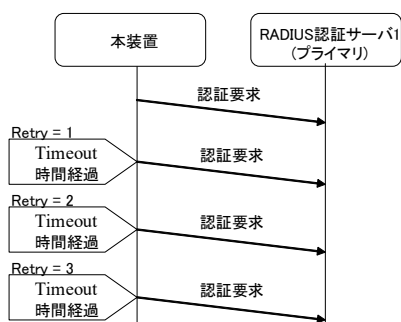
図 2-12 RADIUS 認証サーバーからの応答がない場合
