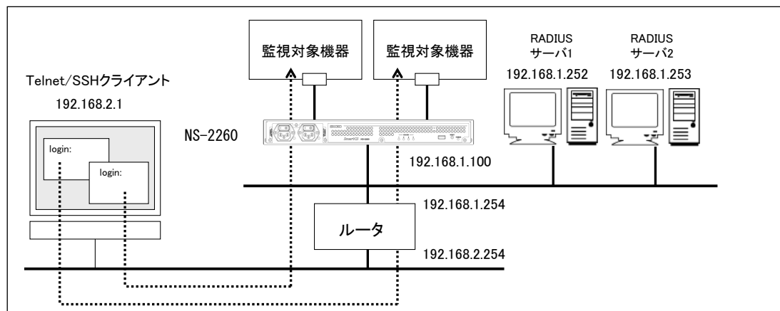
図 4-14 RADIUS 認証機能/RADIUS アカウント機能 (基本構成)
