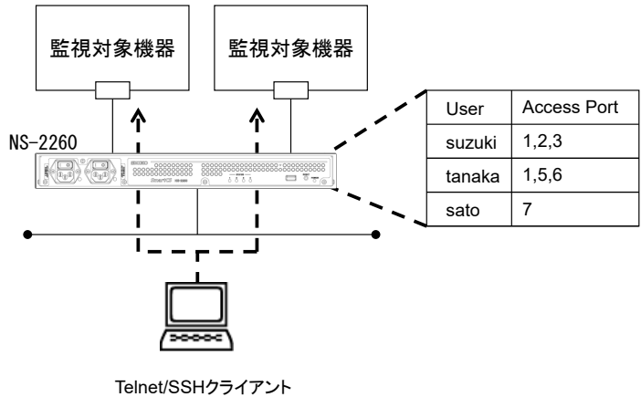
図 2-7 ポートユーザーのシリアルポートアクセス制限
