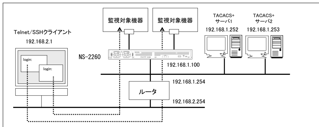
図 4-18 TACACS+機能 (アクセスグルーピング)
