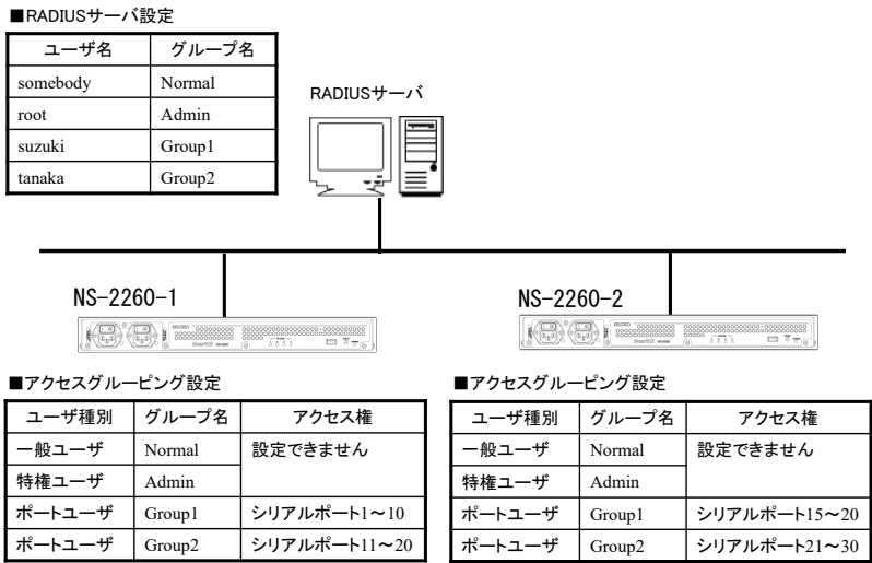
図 2-16 ユーザーグループの識別とシリアルポートのアクセス制限 (アクセスグルーピング)
