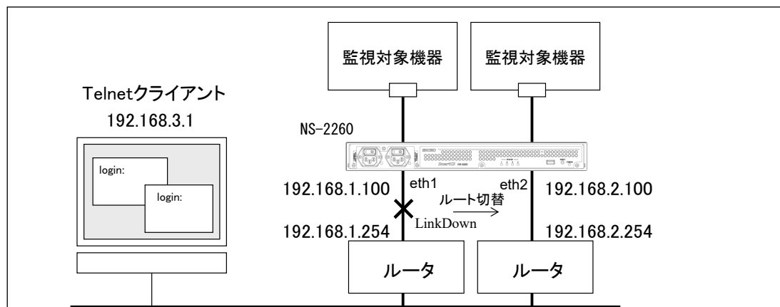
図 4-19 LAN 冗長構成 (2つの LAN ポートを異なるセグメントで利用)
