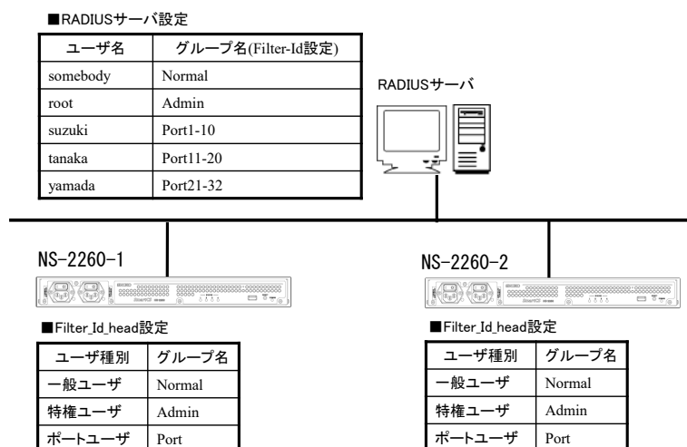
図 4-1 ユーザーグループの識別とシリアルポートのアクセス制限 (filter_id_head)
