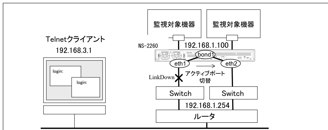
図 4-20 LAN 冗長構成 (ボンディング機能)
