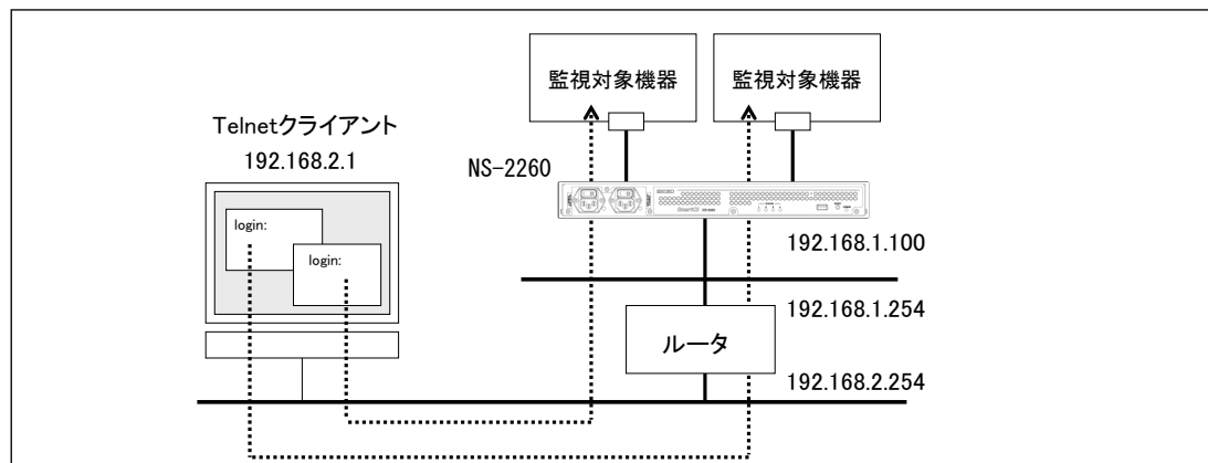
図 4-13 ポートセレクト機能 (ポートサーバーのセレクトモード)
