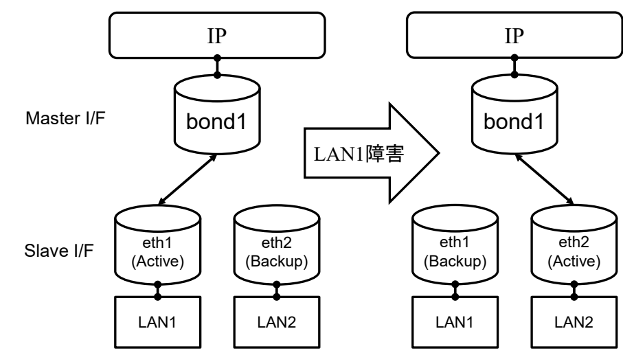
図 2-24 ボンディング機能
