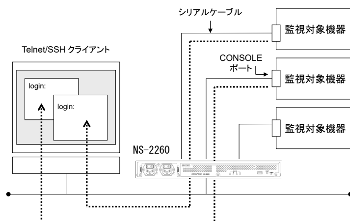
図 1-2 CONSOLE ポートの集約
