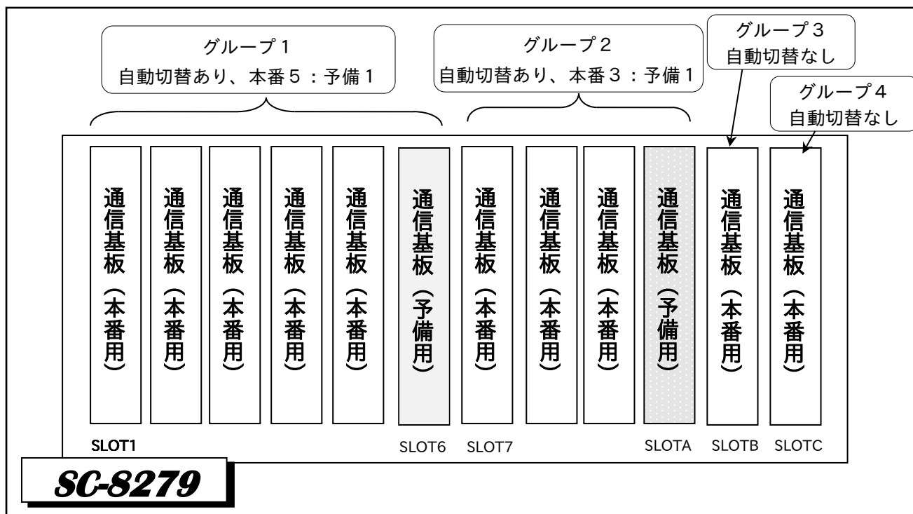
図2. 3 UST設定例
