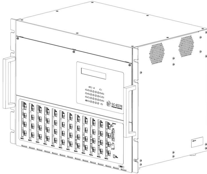
図 1. 6 前方図
