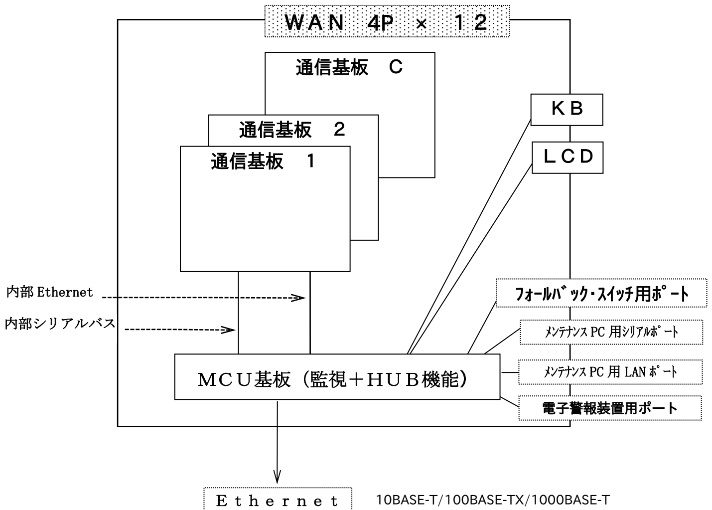
図 1. 5 UST構成
