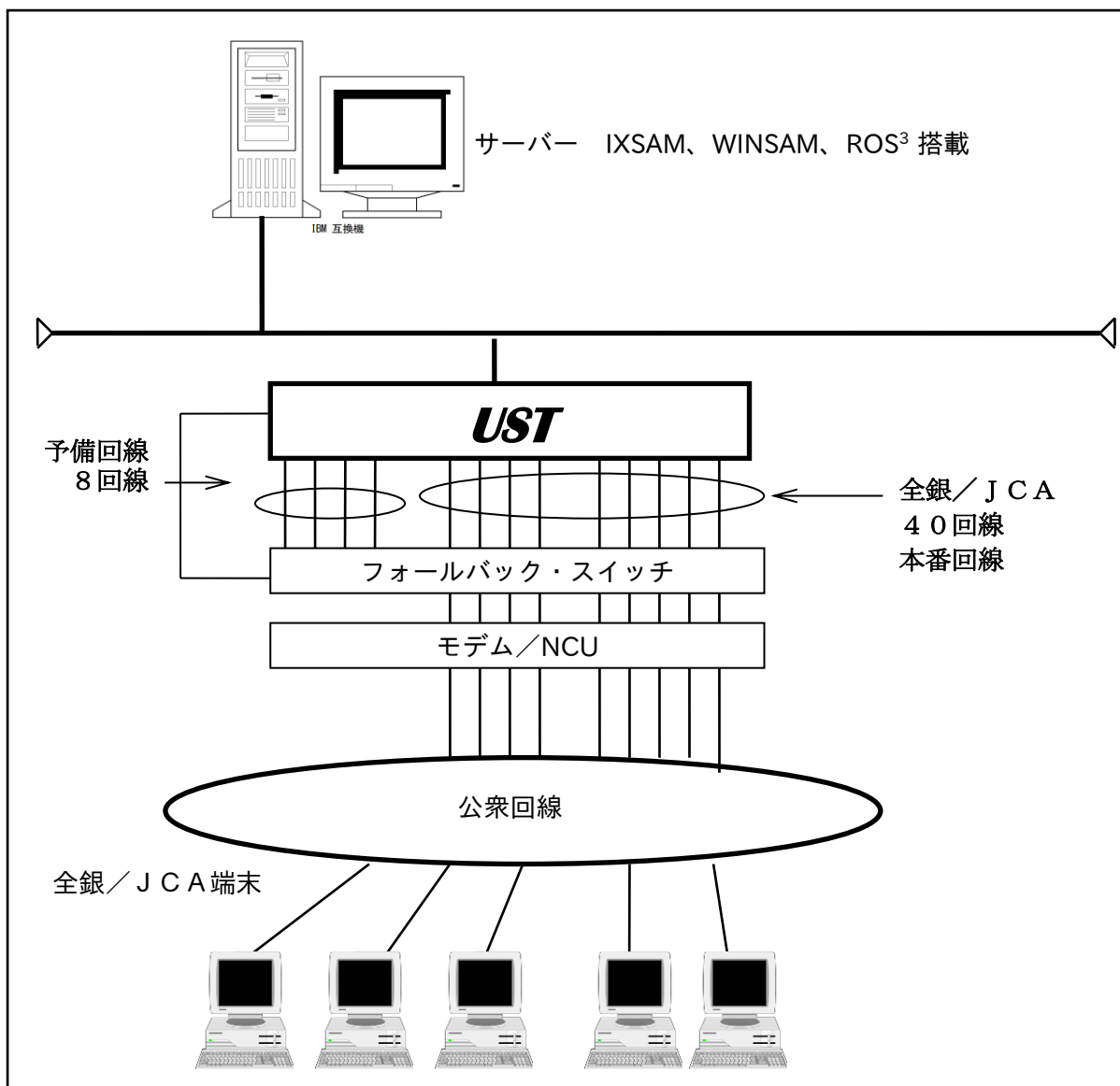
図 1. 4 接続例
