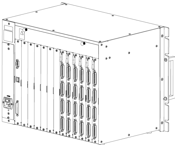
図 1. 7 後方図
