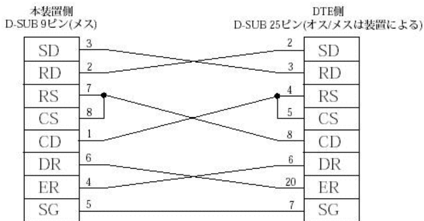
図3-2 9ピン-9ピンヌルモデムケーブル結線図(仕様1)
