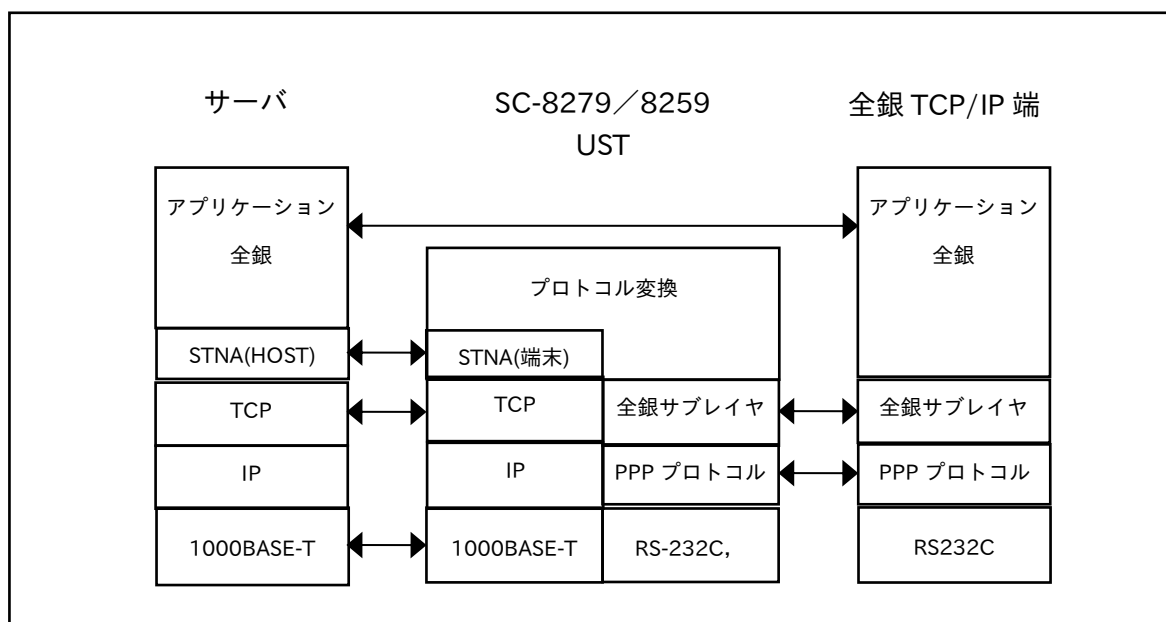
図 1. 3 プロトコル構成(全銀 TCP/IP 接続時)
